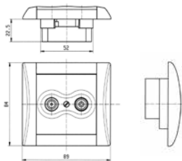
zásuvka TV+R
