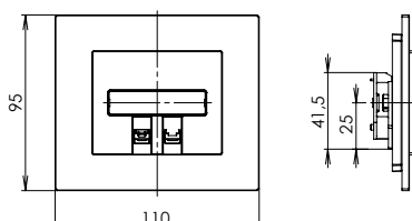
Zásuvka telefonní
