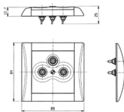
zásuvka AUDIO-VIDEO
