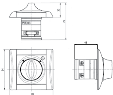
žaluziový ovladač
