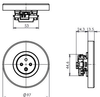
ZÁSUVKA JEDNONÁSOBNÁ
