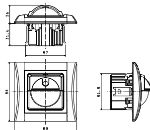
pohybové čidlo
