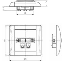
zásuvka telefonní
