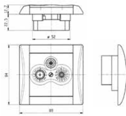
zásuvka TV+R+SAT
