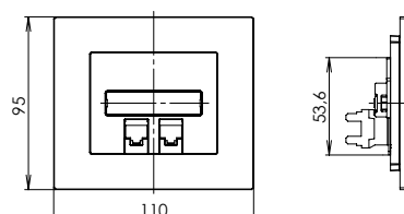
Zásuvka komunikační
