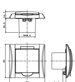
zásuvka vysavačová
