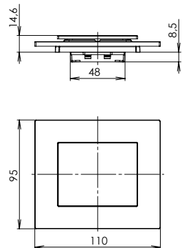
Záslepka
